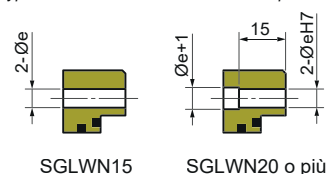
Modello con foro di fissaggio e specifiche dei fori Type with dowel hole and dowel hole specification
