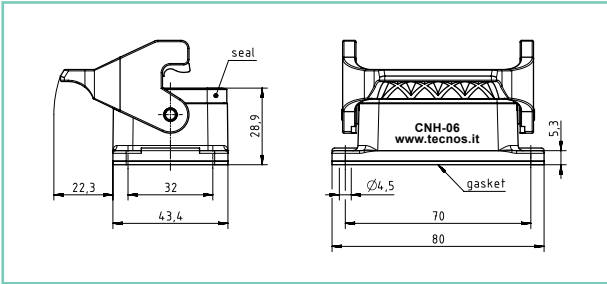
6 POLI Codice: CNH-06
