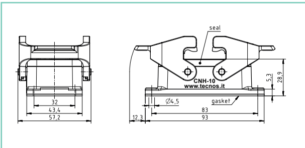
10 POLI Codice: CNH-10
