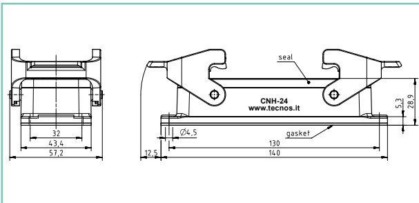
24 POLI Codice: CNH-24
