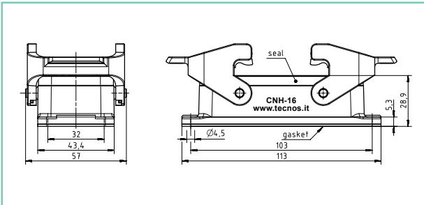
16 POLI Codice: CNH-16
